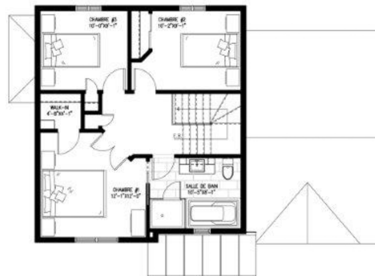
Plan Étage +/- 24'-0 x +/- 27'-0 (environ 638 pc / 59,3 mc)
