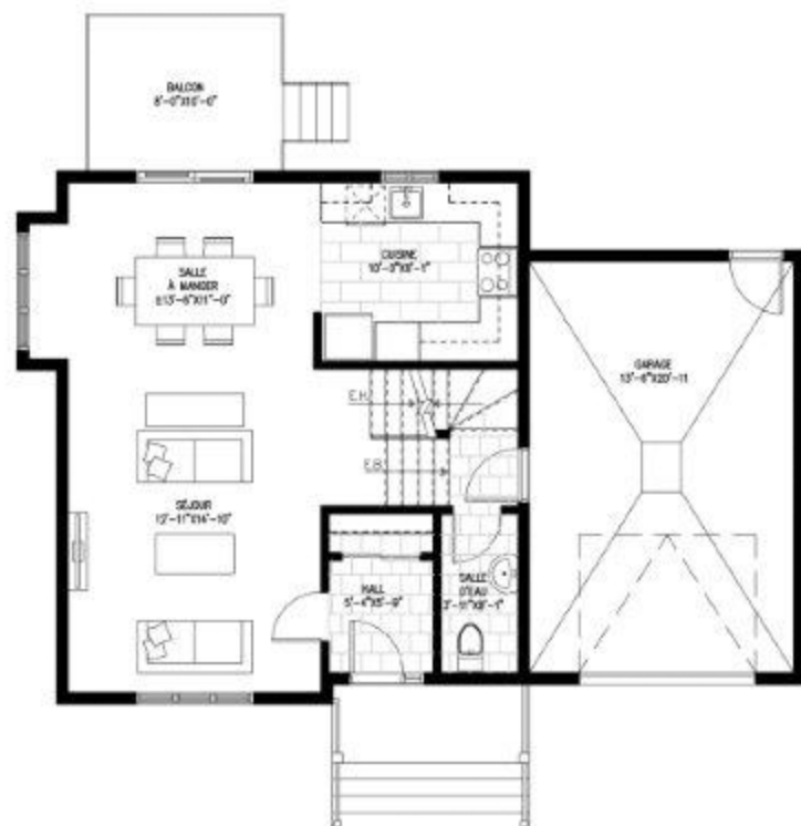
Plan Rez-de-chaussée +/- 24'-0 x +/- 27'-0 (environ 654 pc / 60,8 mc) Garage non inclus
